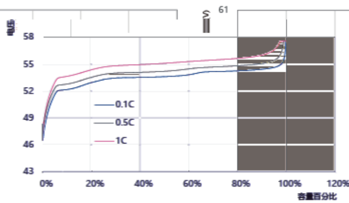
不同倍率下的充电曲线 (25°C)
