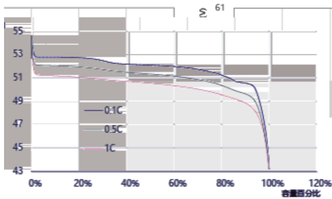
不同倍率下放电曲线 (25°C)
