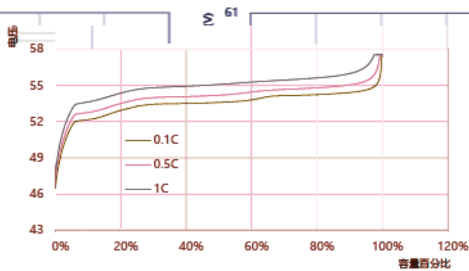
不同倍率下的充电曲线 (25°C)
